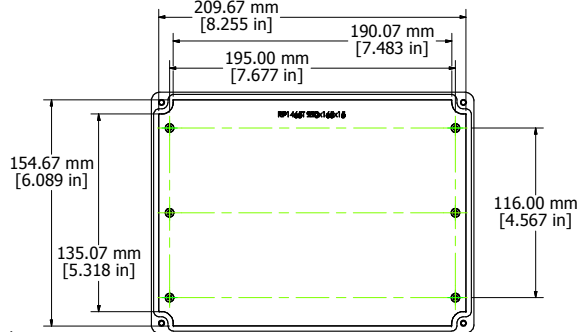
LID - INSIDE
