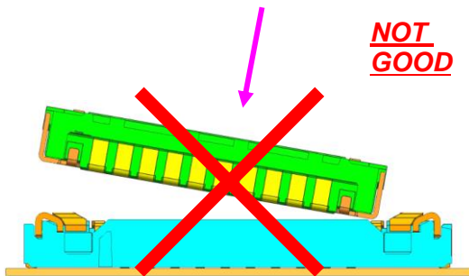
コネクタ斜め嵌合 Mating with angle (Wrong Handling)
